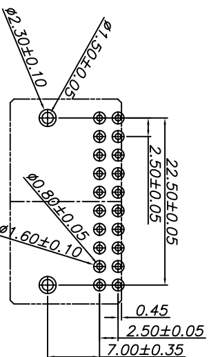
P.C.B. LAYOUT
